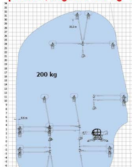
Rotazione su stabilizzatori compl. sfilati con cestello a pendolo rotante 3D positivo / negativo 200 kg - 2 persone
